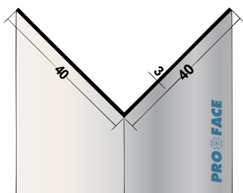
Proface® CORNEQ CQ400-A
